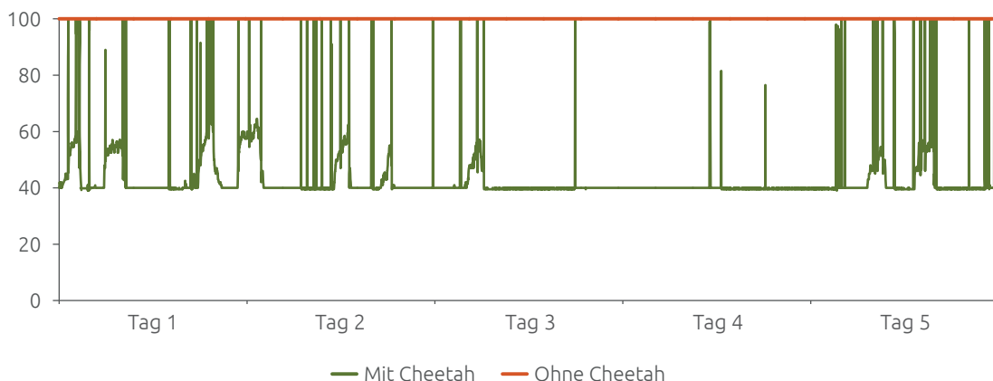
Park Inn Lille: Motordrehzahl mit und ohne Cheetah (in %)
